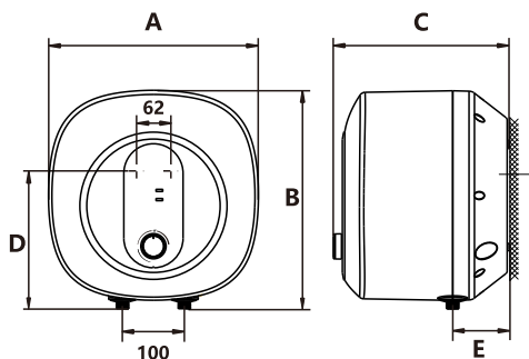
Изведба над мијалник
