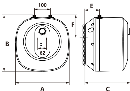
Изведба под мијалник
