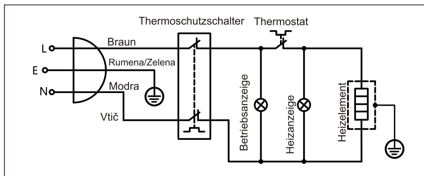
Anschlussplan
