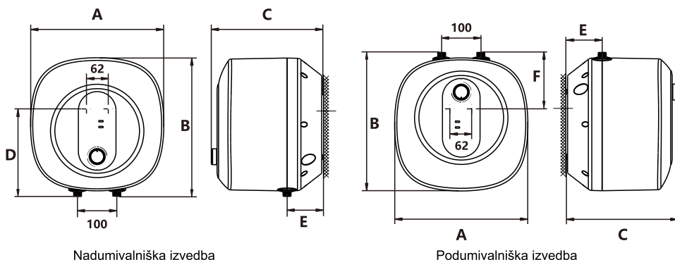
Nadumivalniška izvedba
